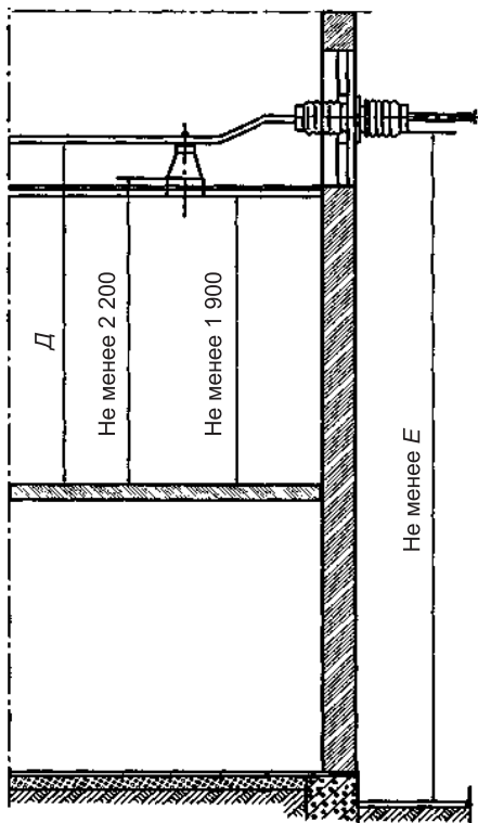
Рисунок 6.2.17 – Наименьшие расстояния от пола до неогражденных незащищенных токоведущих частей и до нижней кромки фарфора изолятора и высота прохода в ЗРУ. Наименьшее расстояние от земли до неогражденных линейных выводов из ЗРУ вне территории ОРУ и при отсутствии проезда транспорта под выводами
